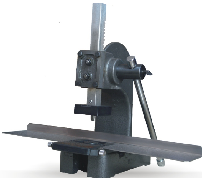
Praska do samodzielnego montażu przelotek, wycinania otworów.
