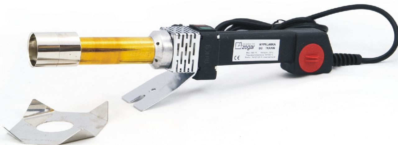
Wypalarka do wypalania otworów w tkaninie, zaopatrzona w dwie zmienne głowice wymienne w zależności od przekroju przelotki.
